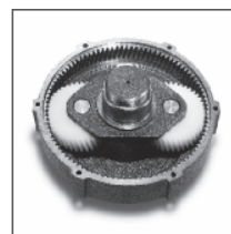
Riduttore ad ingranaggi satelliti e planetario in bagno d'olio
